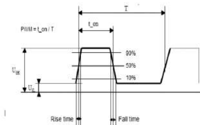
Рис. 4 Форма волны ШИМ
