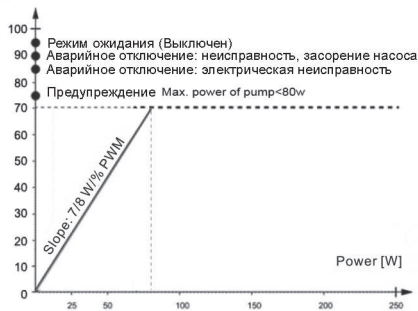
Рис 8. Логика сигнала обратной связи ШИМ
